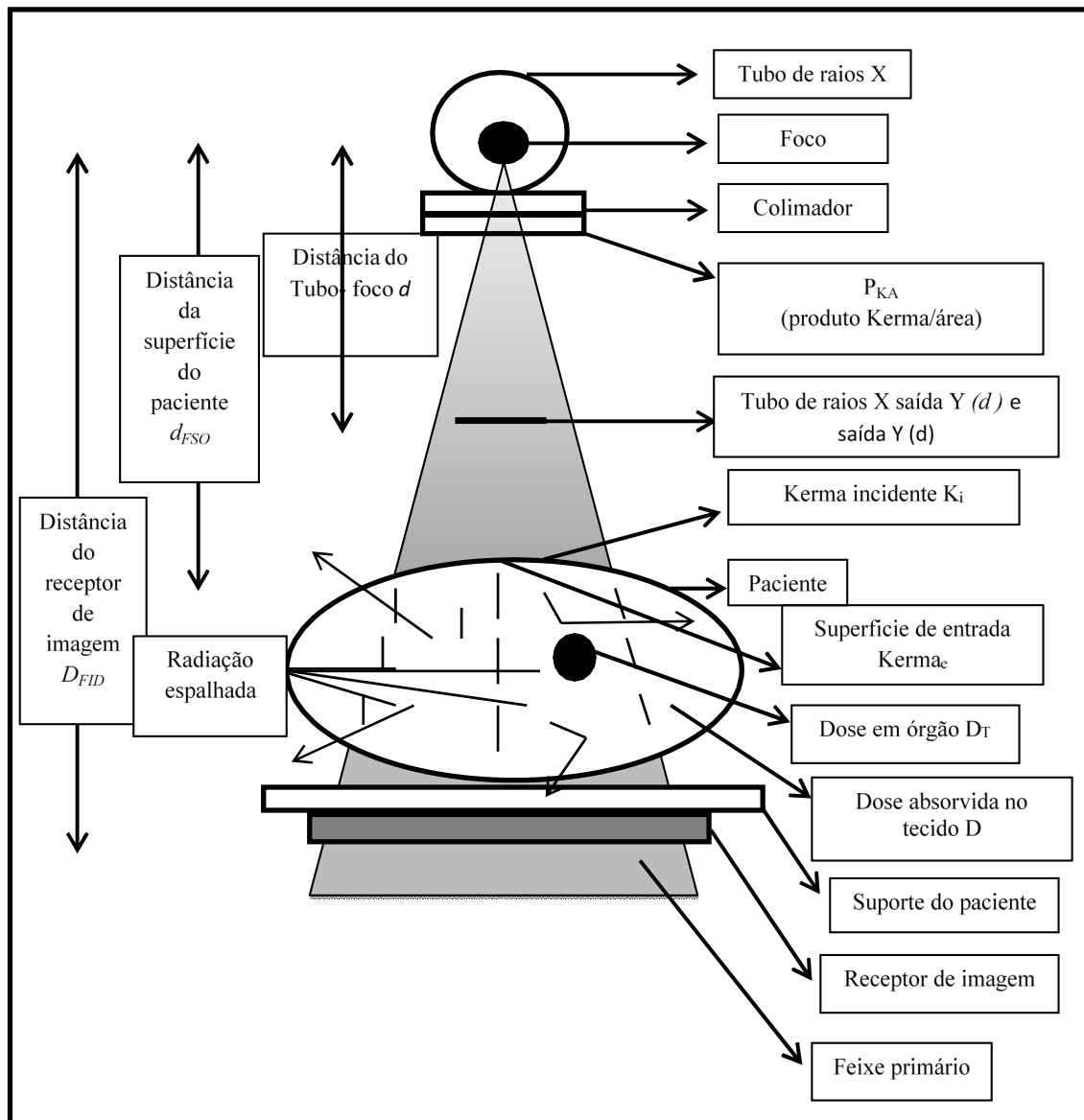
Figura 9 - Grandezas de interesse para estimativa das doses em pacientes e para caracterização do equipamento de raios
